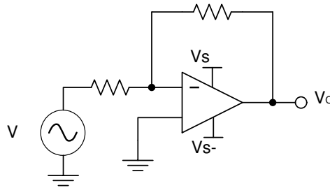
図 9-1. アプリケーション回路図
