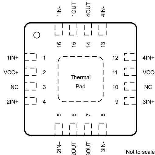
図 4-3. RTE パッケージ 16 ピン WQFN (上面図)
