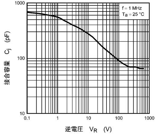
図 9.4 C_j - V_R
