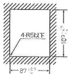
パネルカット寸法図
