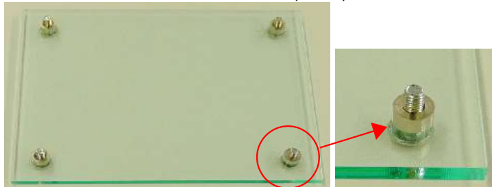
②アクリル板の下から「トラスネジ」を通しアクリル板の上から「丸型スペーサー」をネジに通します(4カ所)
