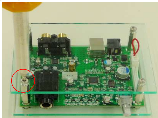
④もう1枚のアクリル板を乗せて「六角穴つきネジ」で固定します(4カ所)
