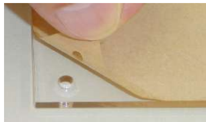
②アクリル板の下から「トラスネジ」を通しアクリル板の上から「丸型スペーサー」をネジに通します(4カ所)
