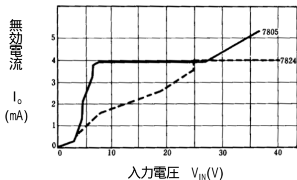
NJM7805/24 無効電流特性例 ( T_j = 25 )
