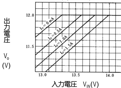
NJM7812 入出力間電位差特性例 ( T_j = 25 )
