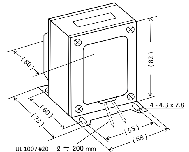
外形寸法図
