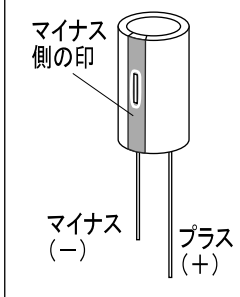
電解コンデンサ
